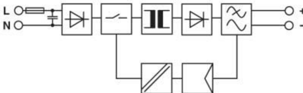
Schéma fonctionnel
