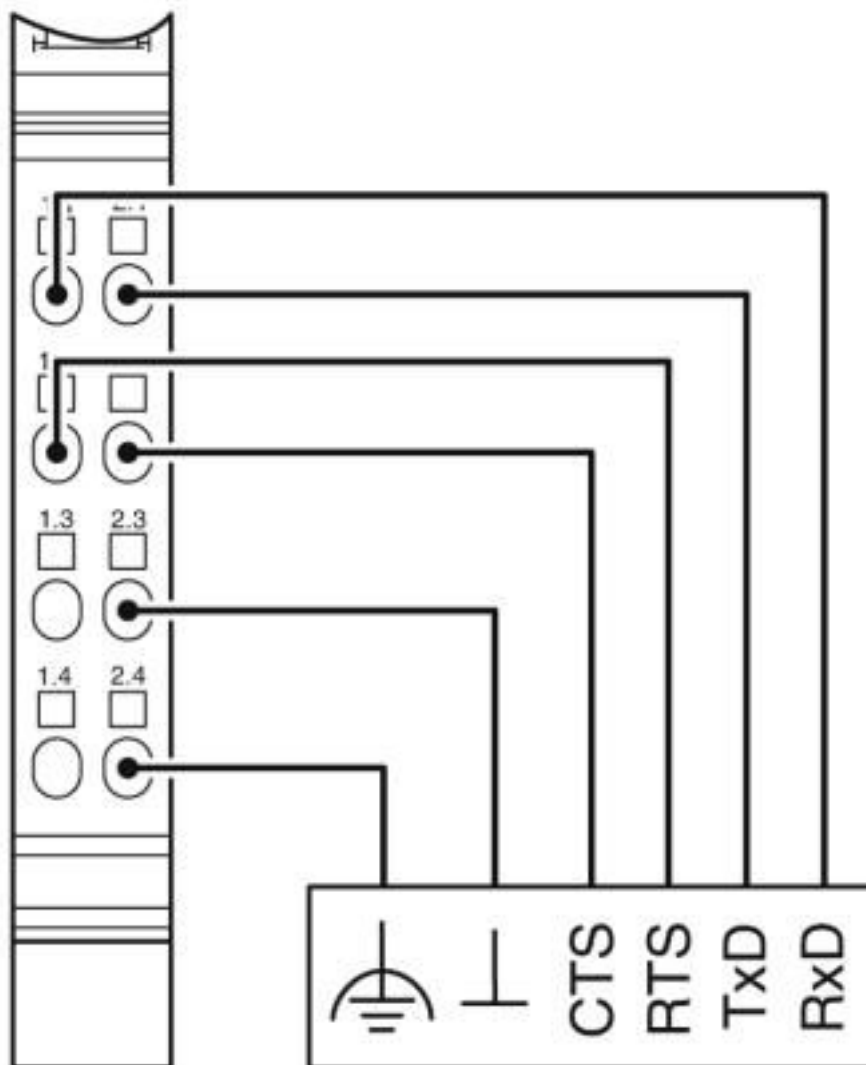
Câblage d'interface RS-232 : Handshake à quatre fils
