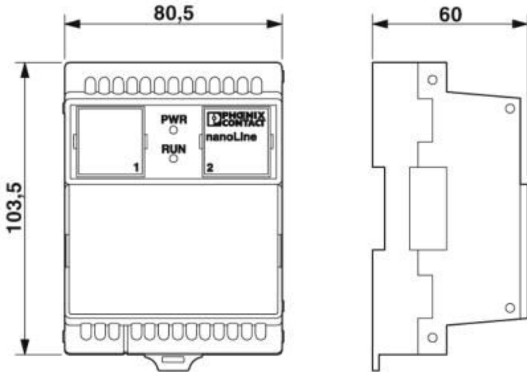
Dessin coté
