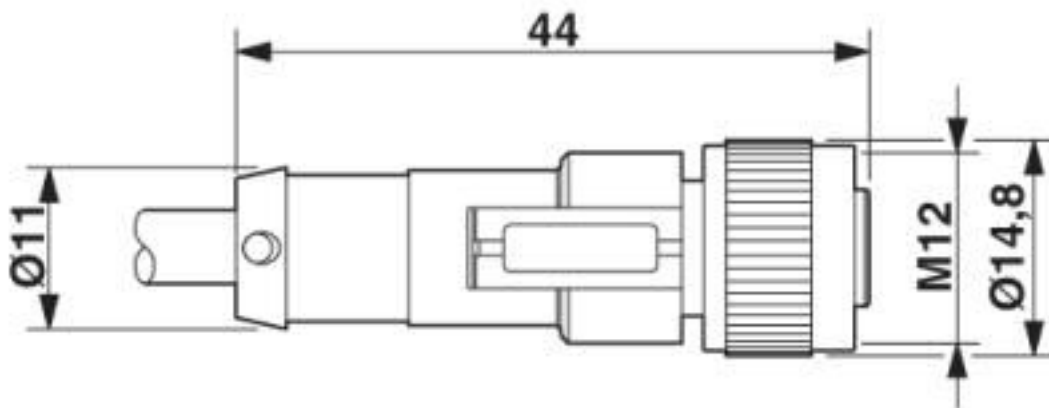
Connecteur femelle M12 x 1, droit
