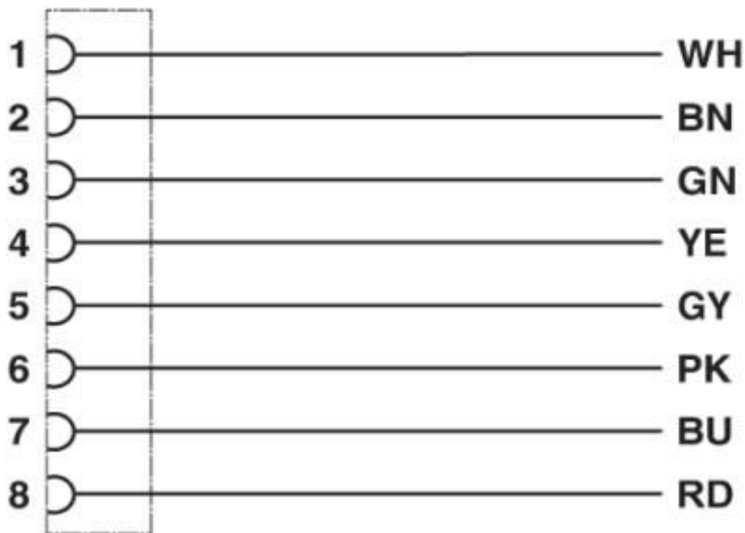
Affectation des contacts du connecteur femelle M12
